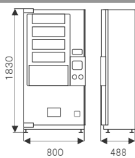
外形寸法図(単位:mm)
