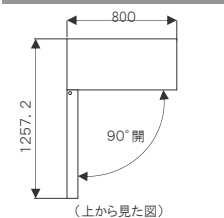
扉開放図(単位:mm)
