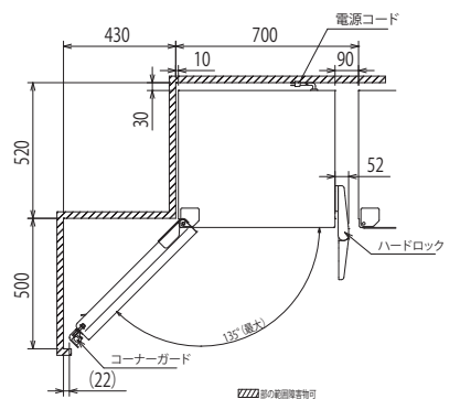
上面設置寸法図(単位:mm)
