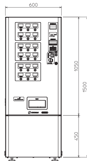
正面図
